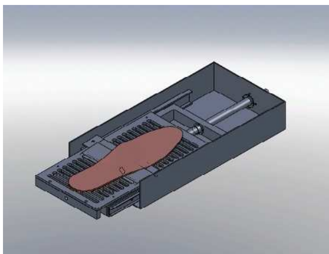
Рис. 5 – Отрезное устройство со стелькой-заготовкой
